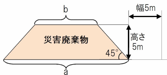
横断面図
