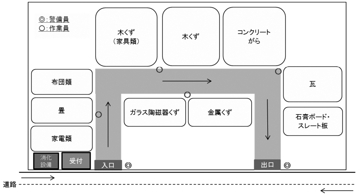
図 6－7 仮置場の分別配置の例
