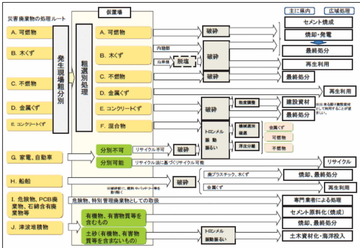
図 6-5 標準的な処理フロー
