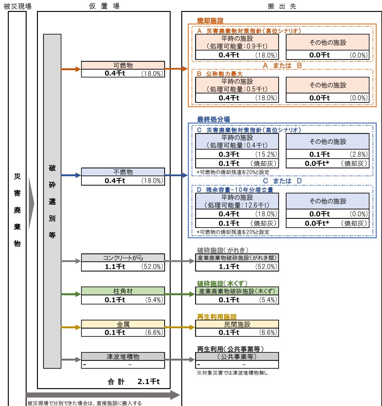
図6-4 十勝沖地震の災害廃棄物処理フロー(例)
