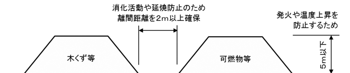
図 6－8 理想的な仮置場の廃棄物堆積状況
